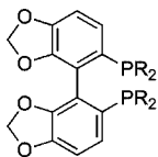
Segphos, R = Ph 8
